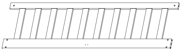
4 Außenwand 2x
