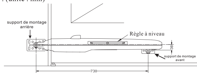
Fig. 6 : (unité : mm)
