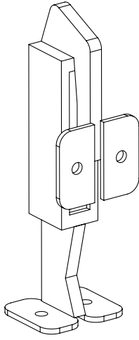
H25 - Hochklappscharnier
