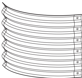
P2 Eckteil, oben 4x
