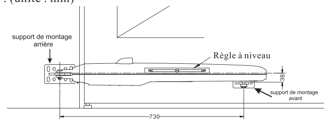
Fig. 6 : (unité : mm)
