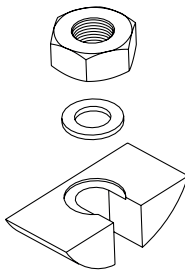
C68 - Halbmondbeschlag
