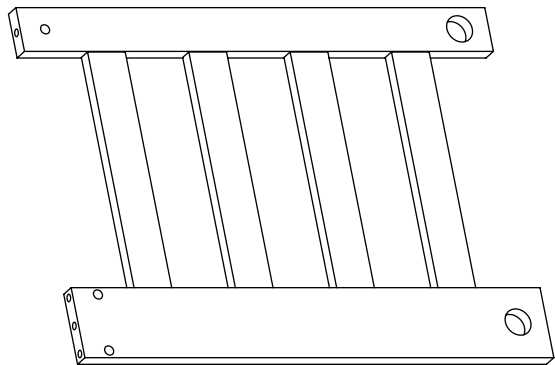
7 Seitenwand 2x
