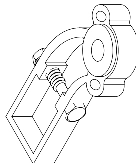
14 Tuchwellenhalter 1x
