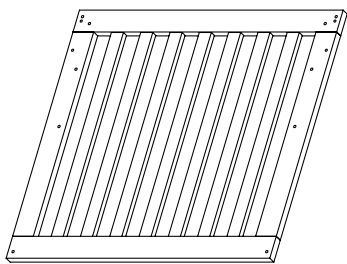
3 Kopf-/Fußteil 2x
