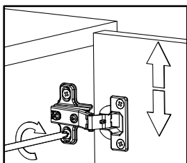
Höhenverstellung Regulacja wysokości Hoogteafstelling Regolazione in Altezza
