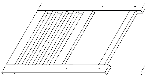
10D Rückenlehne, links 1x
