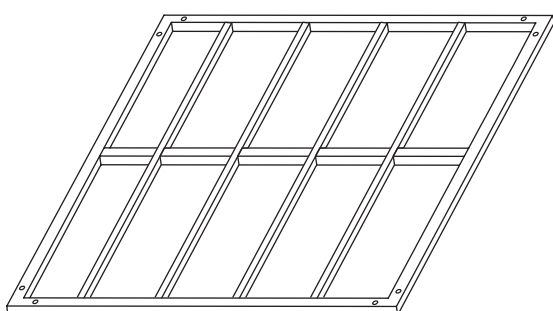
7 Gestell, Liegefläche 2x
