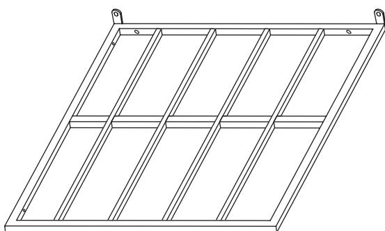
5 Sitzgestell, linker Stuhl 1x
