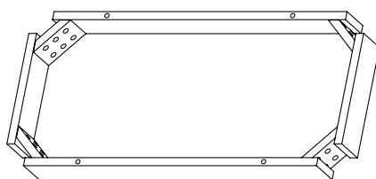
6 Fußrahmen 1x
