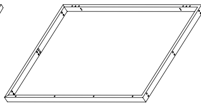
7 Mittelrahmen 1x
