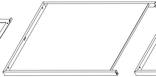
2 Seitenwand, links 1x
