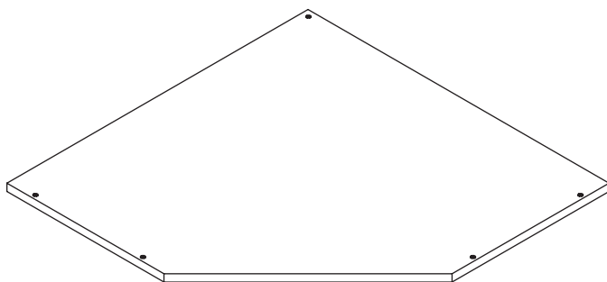
1 Oberboden 1x
