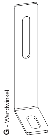
G - Wandwinkel 2x
