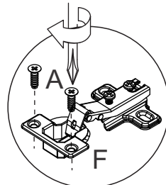
Detalle 20 / Detail 20 Detalhe 20 / Détail 20
