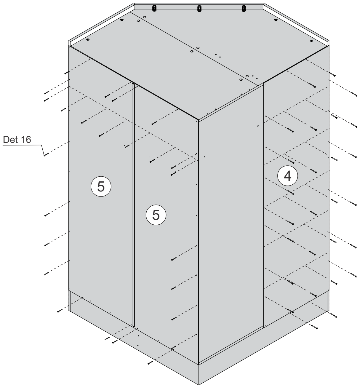
Detalle 16 / Detail 16 Detalhe 16 / Détail 16
