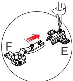
Detalle 19 / Detail 19 Detalhe 19 / Détail 19
