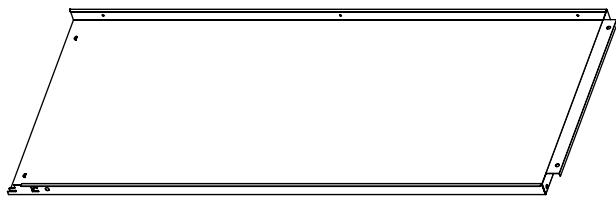
2 Rückwand, links 1x
