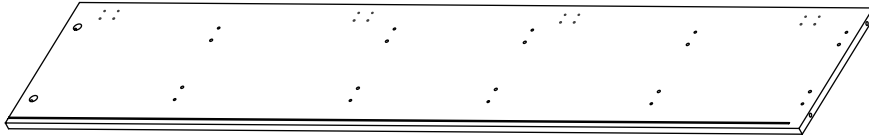
2 Seitenwand, rechts 1x
