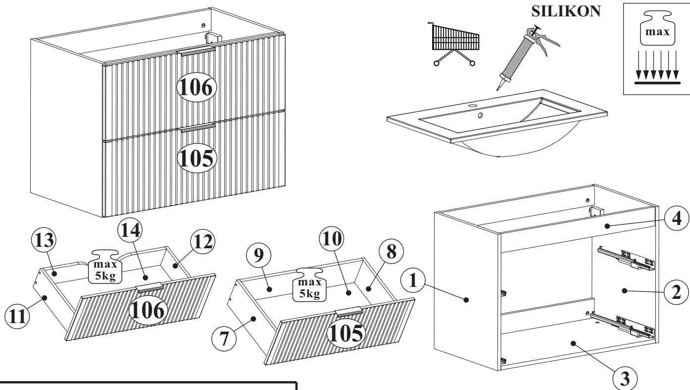
SZAFKA P./UM 2SZ 82-60-D-2S
