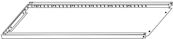
7 Rechte Seitenwand
