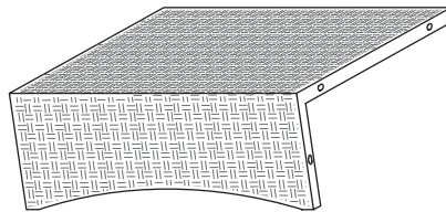
7 Sitzfläche 2x
