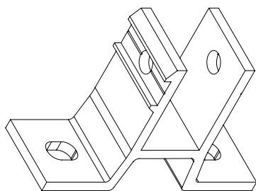
A25 - Wandhalterung
