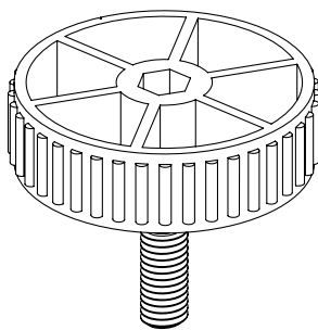
L54 - Fuß
