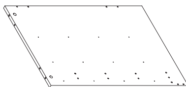
2 Seitenteil 1x
