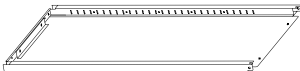
4 Linke Seitenwand
