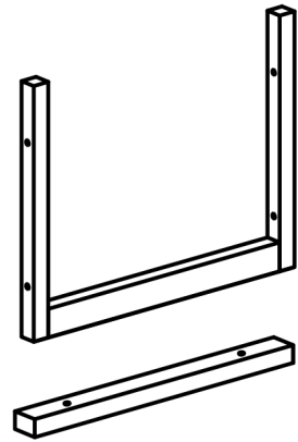
3 Ausgangsrahmen 1x
