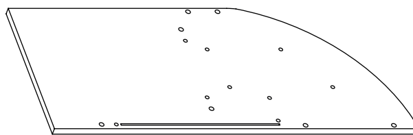
13 Seitenwand, links 1x
