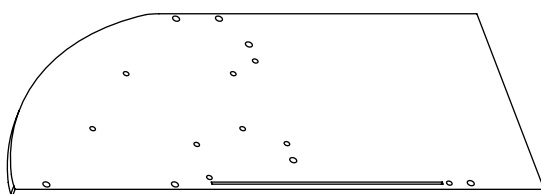
14 Seitenwand, rechts 1x
