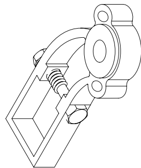
11 Tuchwellenhalter 1x
