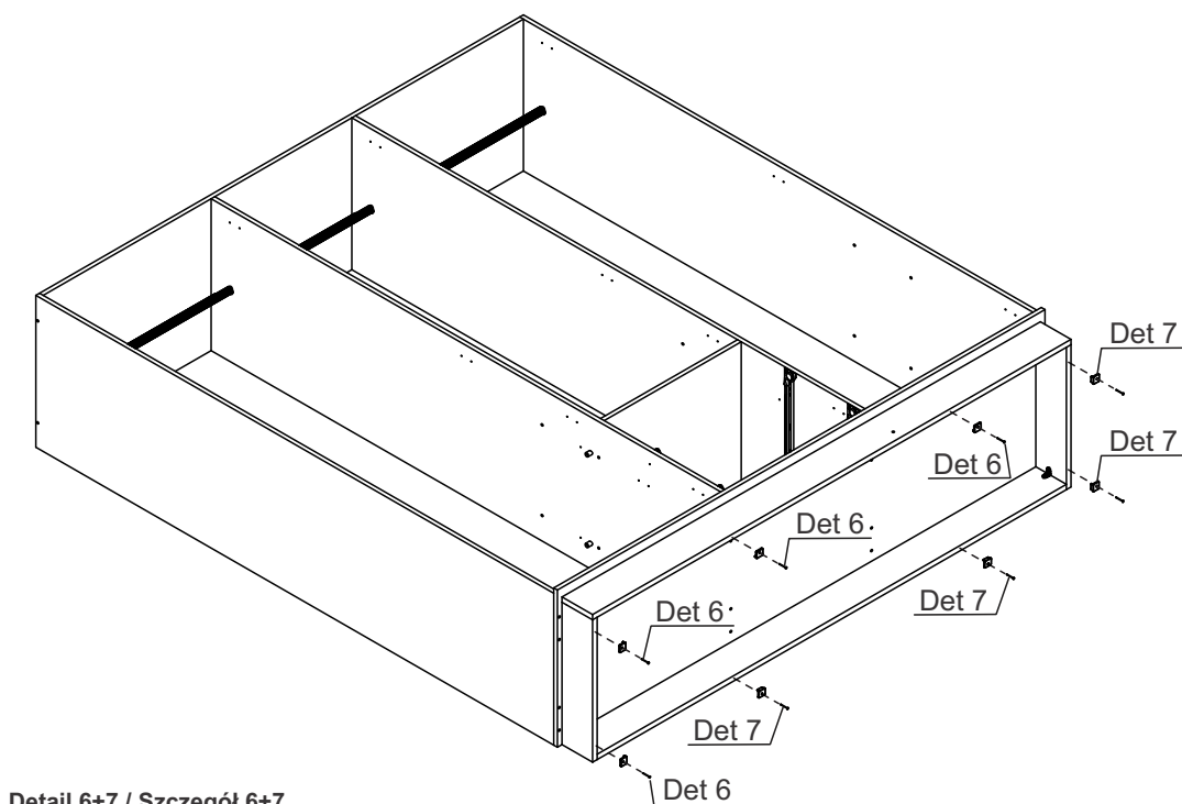
Detail 6+7 / Szczegół 6+7 Detail 6+7 / Dettaglio 6+7
