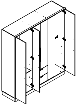
Detail 23 / Szczegół 23 Detail 23 / Dettaglio 23
