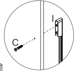
Detail 22 / Szczegół 22 Detail 22 / Dettaglio 22
