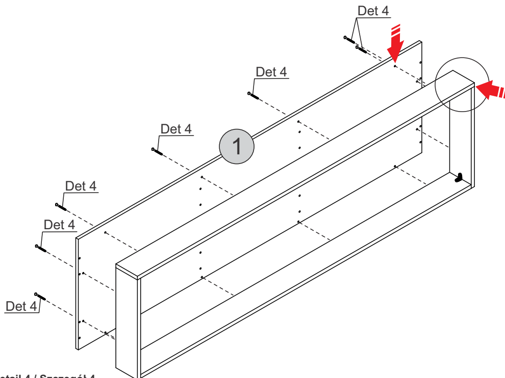
Detail 4 / Szczegół 4 Detail 4 / Dettaglio 4
