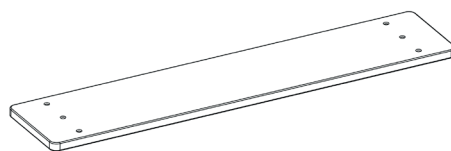
3 Sitzfläche 2x
