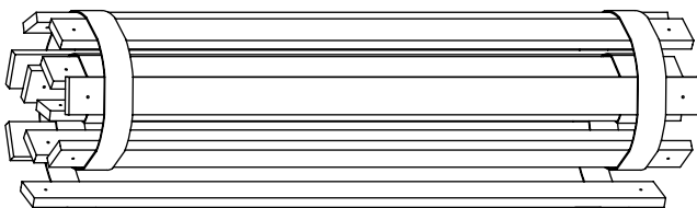
16 Lattenrost 1x
