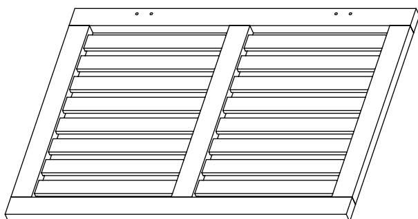
5 Deckel 1x
