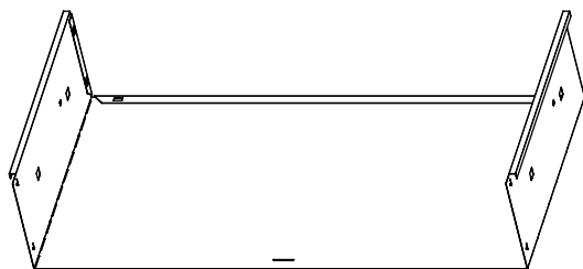
8 Schlade, Korpus 3x
