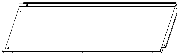
5 Rückwand, rechts 1x
