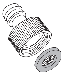
2 Schlauchverschraubung 1x
