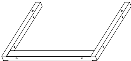
15 Türrahmen 2x
